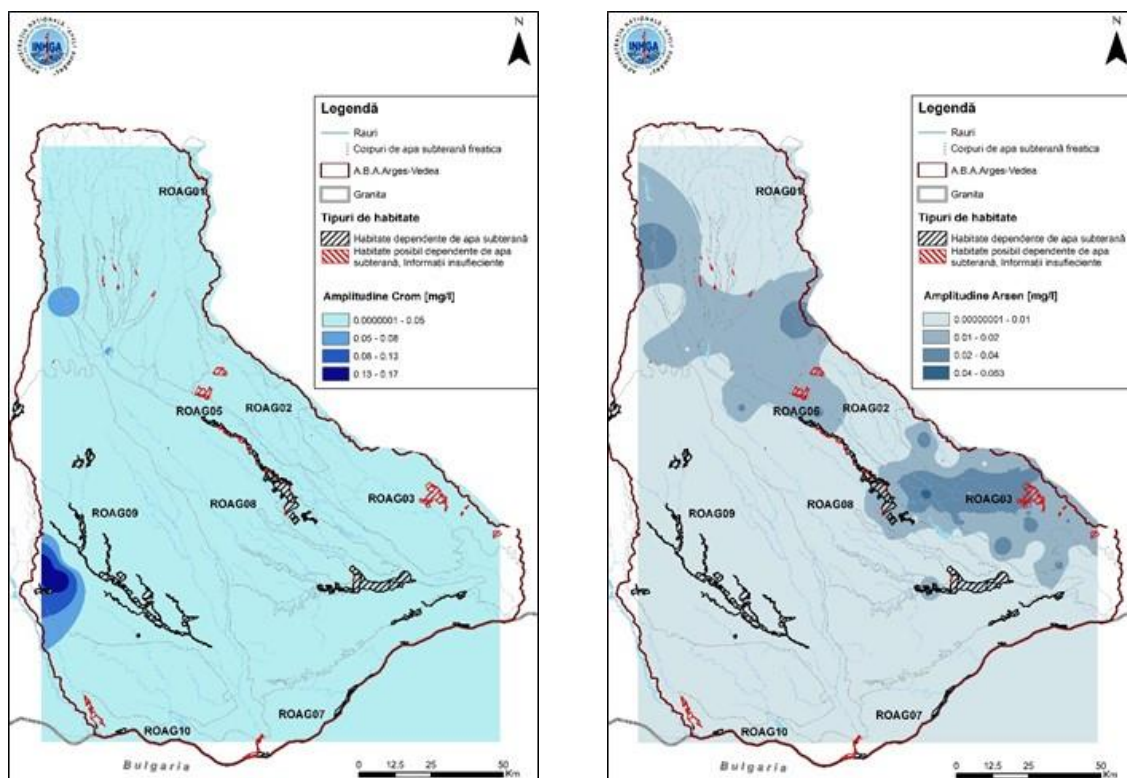
A) B) Figura 4.39 Variația diferenței dintre valoarea maximă și minimă a parametrilor chimici crom (A) și arsen (B) în arealul habitatelor dependente de subterană
