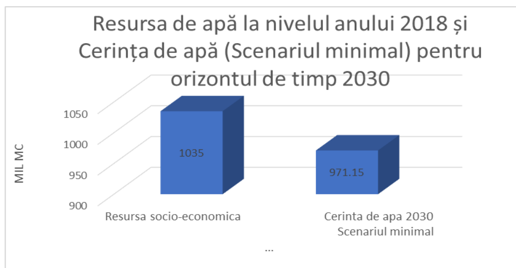
Figura nr. 8.12. Resursa de apă- (anul 2018) și Cerința de apă- (orizontul de timp 2030)
