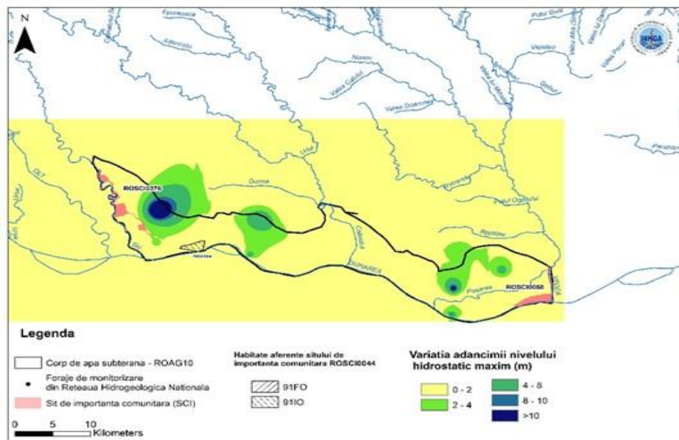
Figura 4.33 Variația adâncimii maxime anuale a nivelului hidrostatic înregistrată în perioada 2000-2017, în fiecare din forajele de monitorizare, în arealul corpului de apă subterană ROAG10
