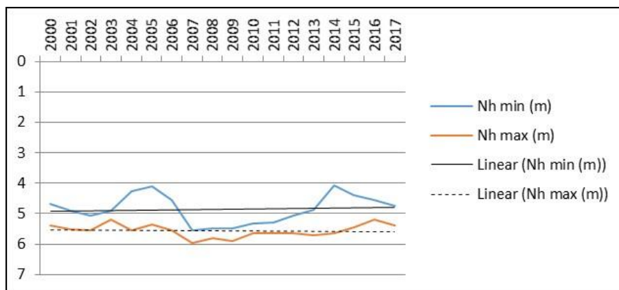
Figura 4.15 Variația adâncimii minime și maxime anuale a nivelului hidrostatic (m) măsurată față de cota terenului, în perioada 2000-2017, în forajul F1 Ionești situat în arealul nord-estic al sitului ROSCI0106 -corpul de apă subterană ROAG05
