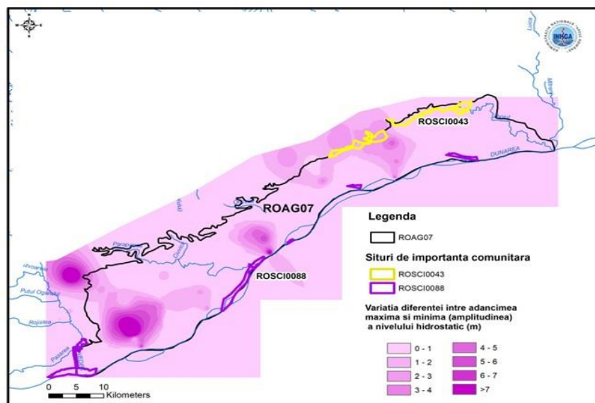
Figura 4.21 Variația amplitudinii adâncimii nivelului hidrostatic în perioada 2000-2017 în zona corpului de apă subterană ROAG07
