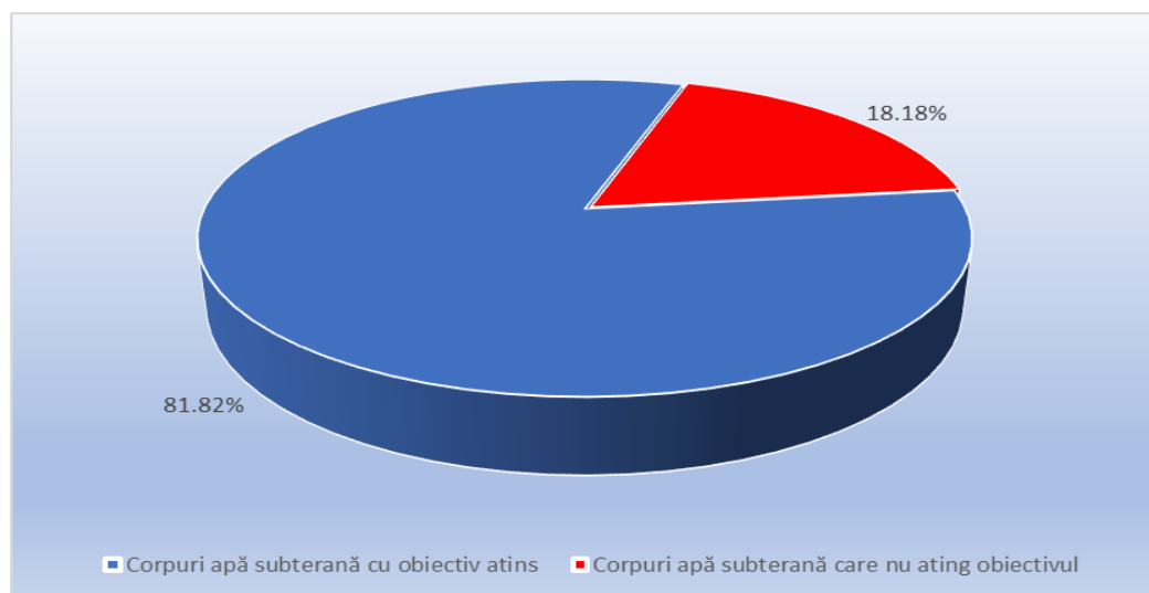
Figura 7.2 Obiectivele de mediu pentru corpurile de apă subterană la nivelul spațiului hidrografic Argeș-Vedea
