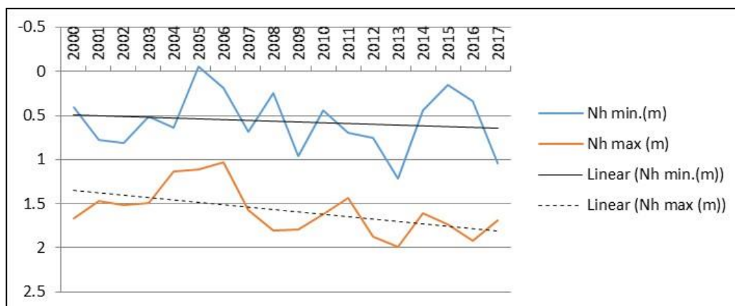
Figura 4.29 Variația adâncimii minimă și maximă anuală a nivelului hidrostatic (m) măsurată față de cota terenului, în perioada 2000 - 2017, în forajul F3 Peretu, situat în apropierea habitatului cu codul 6430 a sitului ROSCI0386, corpul de apă subterană ROAG09
