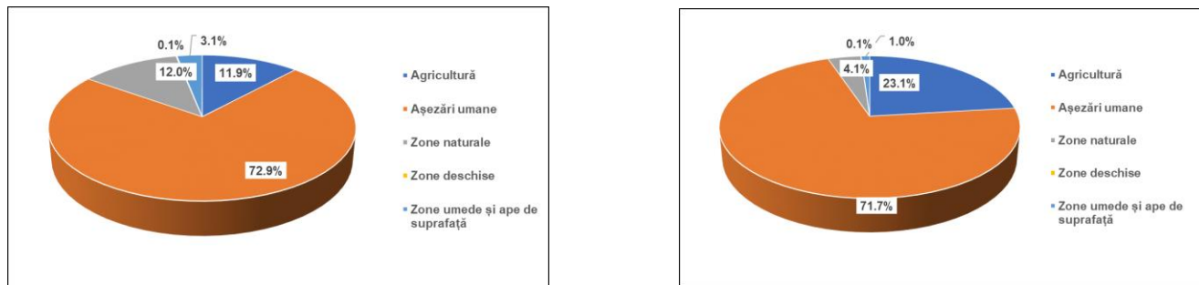
Figura 3.10. Distribuția surselor de emisii în spațiul hidrografic Argeș-Vedea pentru perioada de referință (2015-2018); la stânga sursele pentru azot total, la dreapta sursele pentru fosfor total
