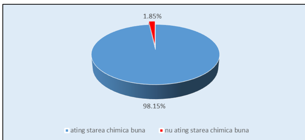
Figura 6.24. Starea chimică a corpurilor de apă naturale (râuri) la nivelul spațiului hidrografic Argeș - Vedea
