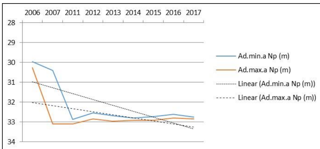
Figura 4.7 Variația adâncimii minime și maxime anuale a nivelului hidrostatic (m) măsurată față de cota terenului, în perioada 2006- 2017, în forajul F1 Cernica situat în zona vestică a sitului ROSCI0308, corpul de apă subterană ROAG03
