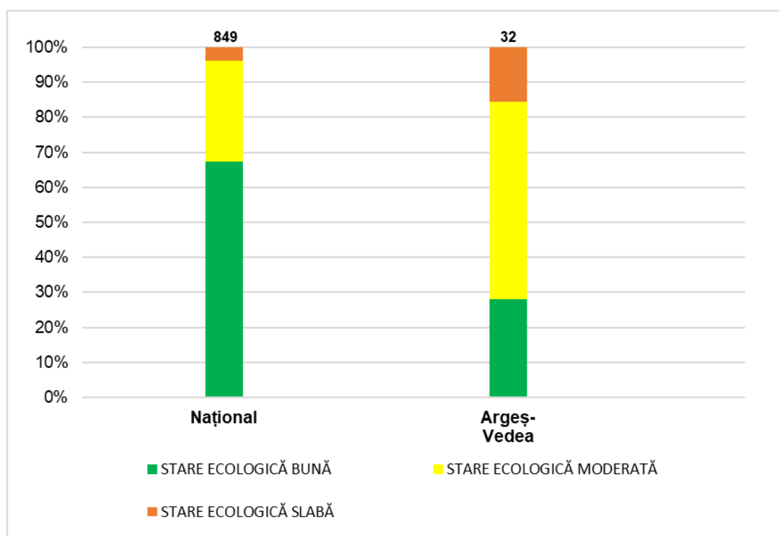
Figura 6.9. Starea ecologică a corpurilor de apă nepermanente - râuri la nivel național și pe spațiul hidrografic Argeș-Vedea
