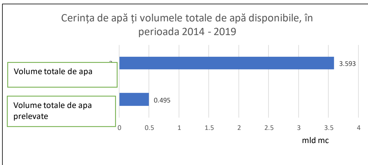
Figura nr. 8.11. Cerința de apă și disponibilul în sursă, în perioada 2014-2019
