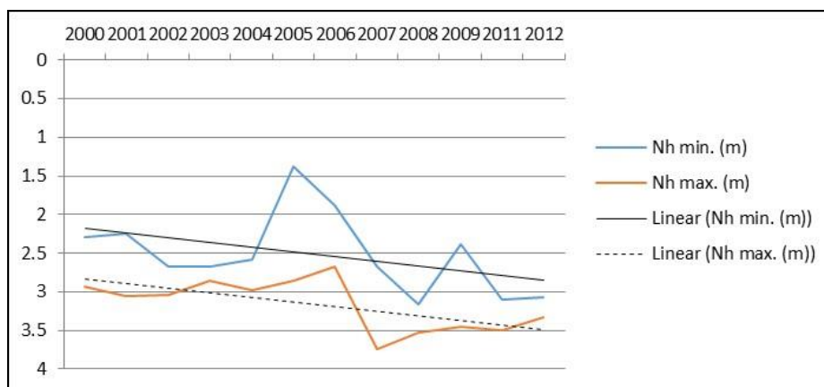
Figura 4.16 Variația adâncimii minime și maxime anuale a nivelului hidrostatic (m) măsurată față de cota terenului, în perioada 2000-2012, în forajul F1 Potlogi situat în partea centrală a sitului ROSCI0106 -corpul de apă subterană ROAG05
