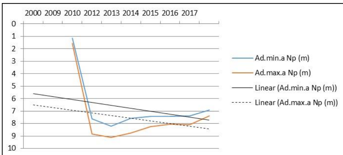
Figura 4.6 Variația adâncimii minime și maxime anuale a nivelului hidrostatic (m) măsurată față de cota terenului, în perioada 2010 - 2017, în forajul F2 Cernica situat în zona vestică a sitului ROSCI0308 (în imediata apropiere de râul Colentina) - corpul de apă subterană ROAG03
