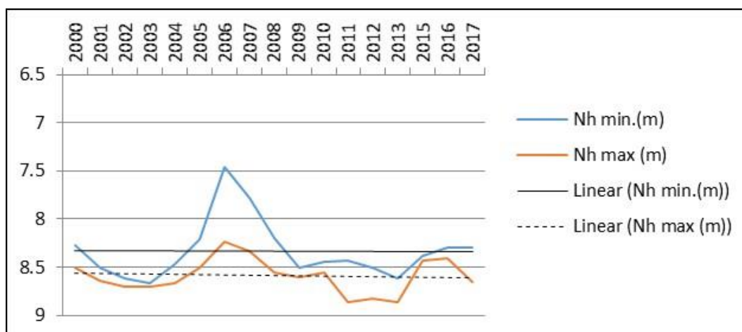
Figura 4.24 Variația adâncimii minime și maxime anuale a nivelului hidrostatic (m) măsurată față de cota terenului, în perioada 2000-2017, în forajul F1 Crevedia Mare ord.II, situat în zona centrală a sitului ROSCI0138, corpul de apă subterană ROAG08
