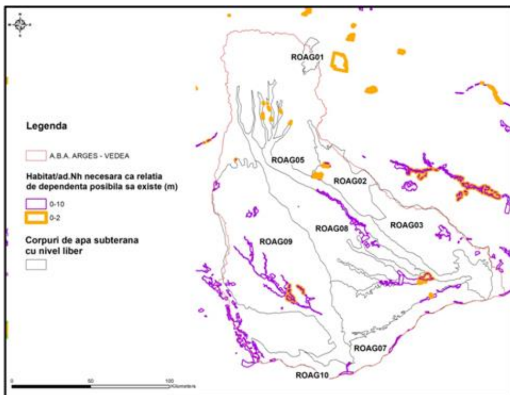
Figura 4.2 Corpurile de apă subterană freatice aferente ABA Argeș - Vedeia și habitatele situate în arealul acestora
