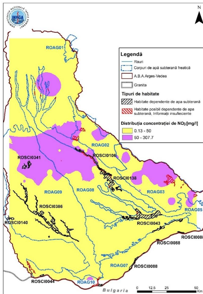
Figura 4.40 Variația concentrației de NO 3 în arealul habitatelor dependente de corpurile de apă subterană ROAG03 și ROAG08 pentru perioada 2014-2017
