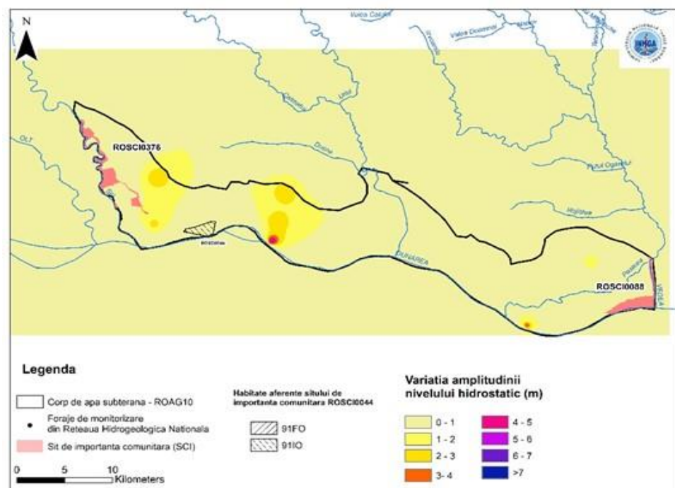
Figura 4.34 Variația amplitudinii adâncimii nivelului hidrostatic în perioada 2000-2017 în zona corpului de apă subterană ROAG10
