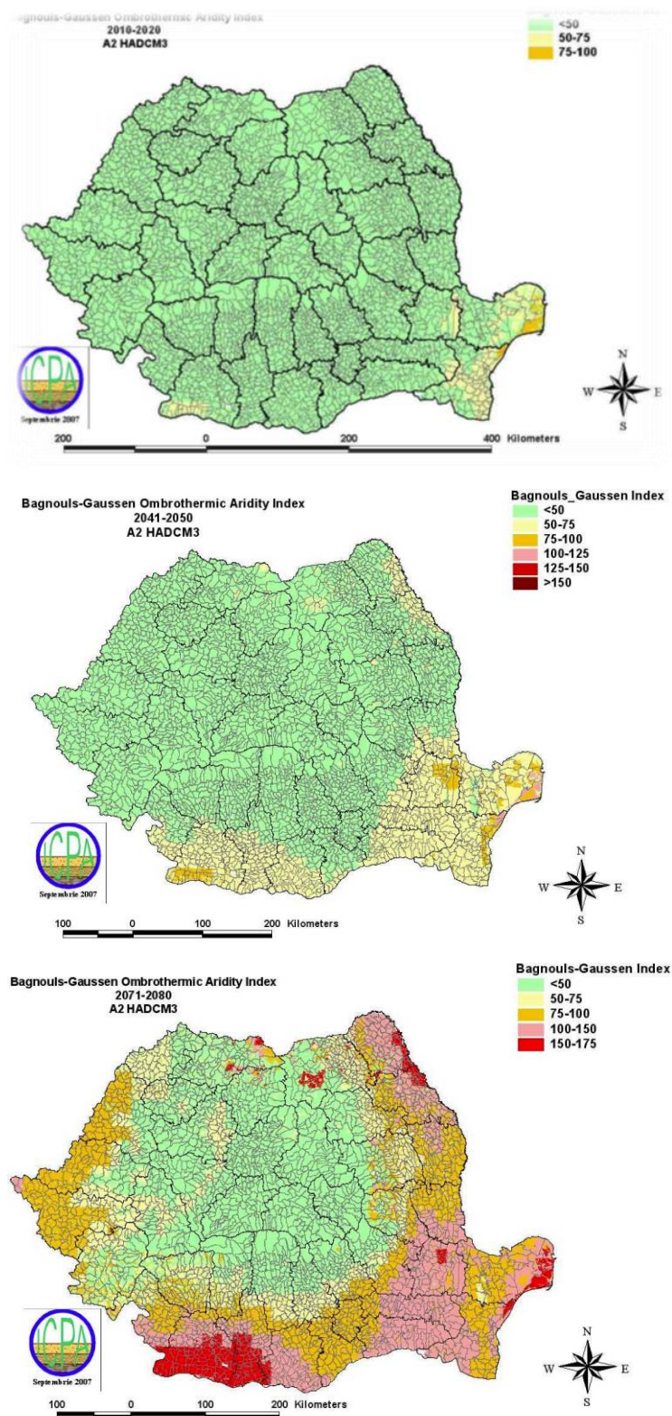
Figura 11.7. Prognoze privind intensitatea fenomenului de secetă pedologică (2010-2080)
