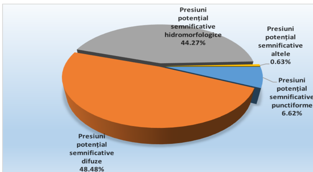
Figura 3.25. Ponderea presiunilor potențial semnificative în spațiul hidrografic Argeș-Vedea
