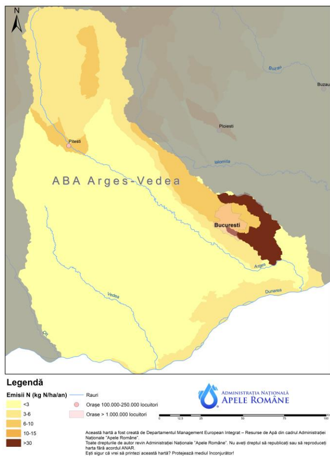
Figura 3.19 Emisia specifică de azot total din surse punctiforme și difuze la nivelul spațiului hidrografic Argeș-Vedea (unități analitice): situația de referință 2015-2018 (stânga) și scenariu de bază 2027 (dreapta)
