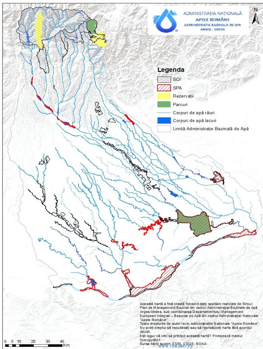
Figura 5.3. Zone destinate pentru protecția habitatelor și speciilor unde apa este un factor important din spațiul hidrografic Argeș-Vedea
