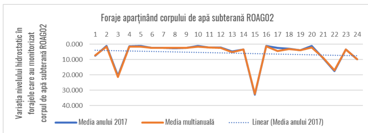
Figura 6.29 Evoluția nivelurilor hidrostatice multianuale (2000-2017) și media anuală în anul 2017 pentru corpul de apă subterană ROAG02
