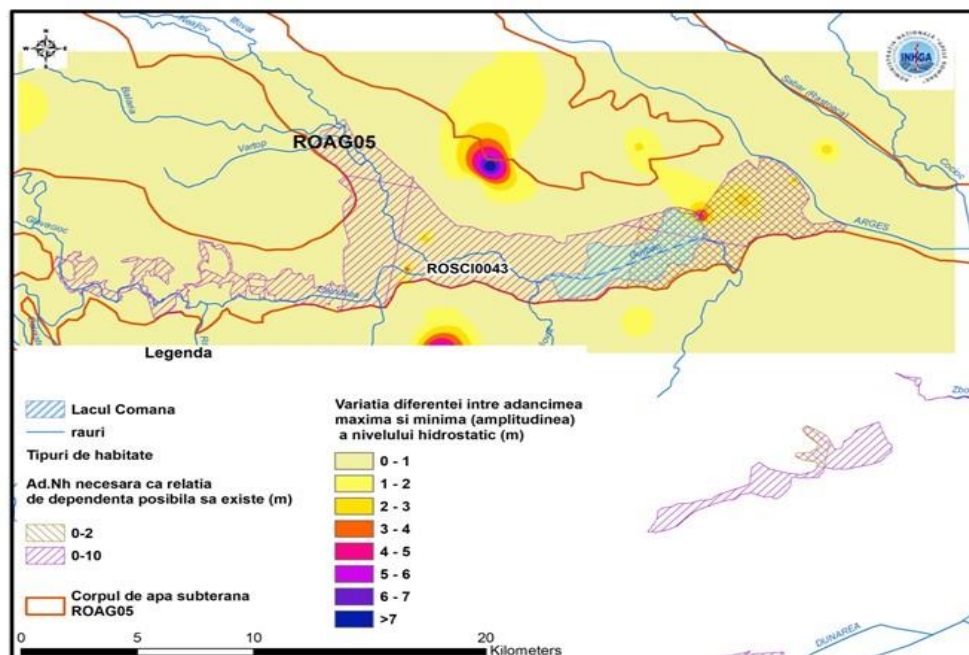
Figura 4.14 Variația amplitudinii adâncimii nivelului hidrostatic în perioada 2000-2017 în zona sitului de importanță comunitară ROSCI0043, corpul de apă subterană ROAG05
