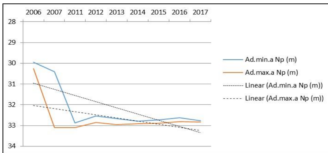
Figura 4.4 Variația adâncimii minime și maxime anuale a nivelului hidrostatic (m) măsurată față de cota terenului, în perioada 2006-2017, în forajul F1 Picior de Munte ord.II situat în zona sud-estică a perimetrului nordic al sitului ROSCI0344, corpul de apă subterană ROAG02
