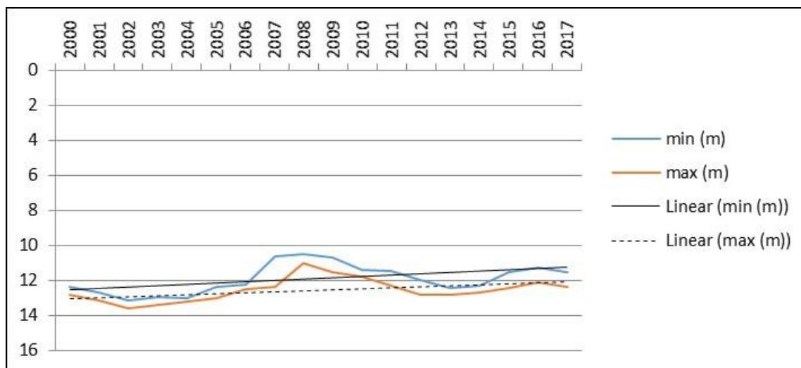
Figura 4.8 Variația adâncimii minime și maxime anuală a nivelului hidrostatic (m) măsurată față de cota terenului, în perioada 2000 - 2017, în forajul F1 Nana Nord ord.II situat în zona nordică a sitului ROSCI0343, corpul de apă subterană ROAG03
