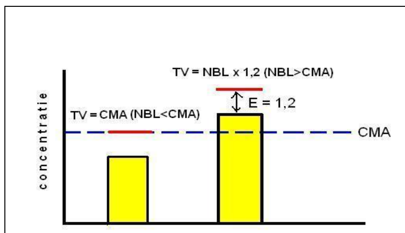
Figura 6.38 Schema de determinare a valorilor prag, funcție de valoarea fondului natural și a concentrației maxime admisibile.
