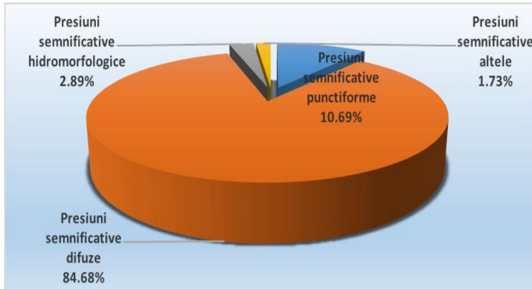
Figura 3.26. Ponderea presiunilor semnificative în spațiul hidrografic Argeș-Vedea
