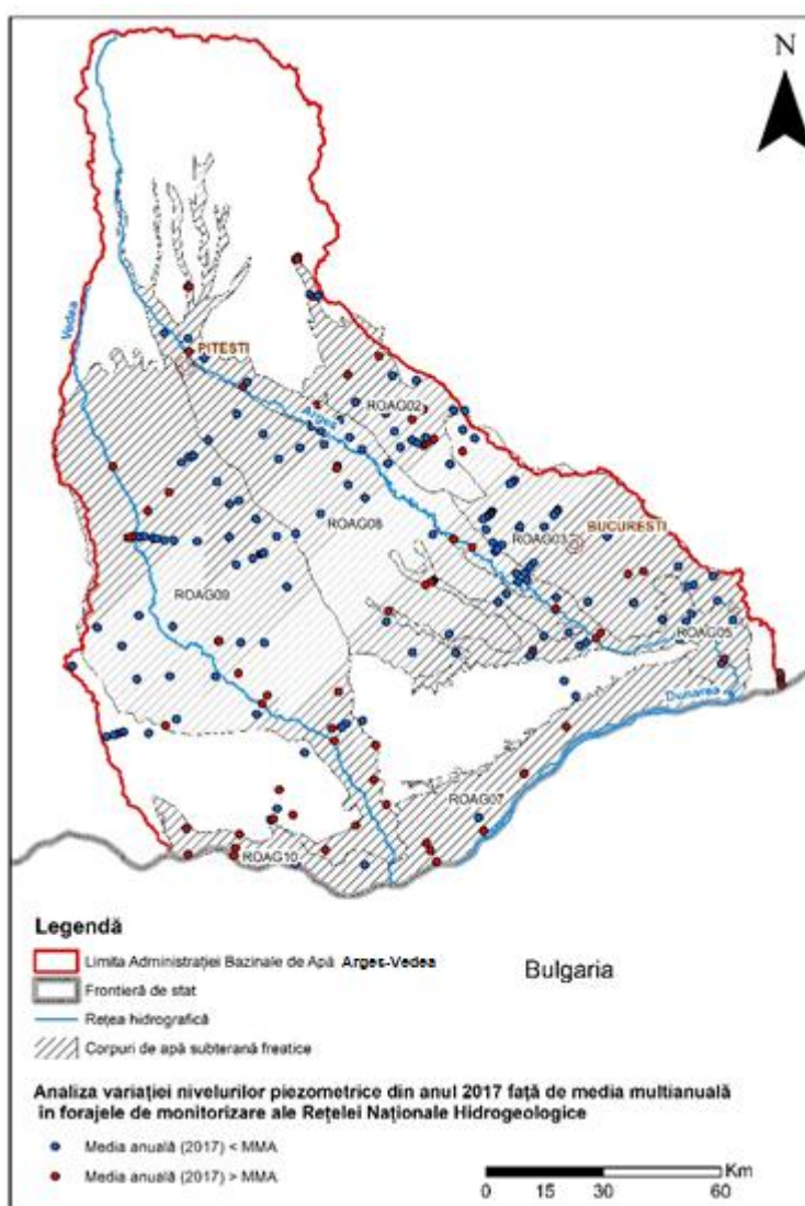
Figura 6.28 Analiza evoluției nivelurilor hidrostatice în forajele de monitorizare cantitativă de la ABA Argeș-Vedea
