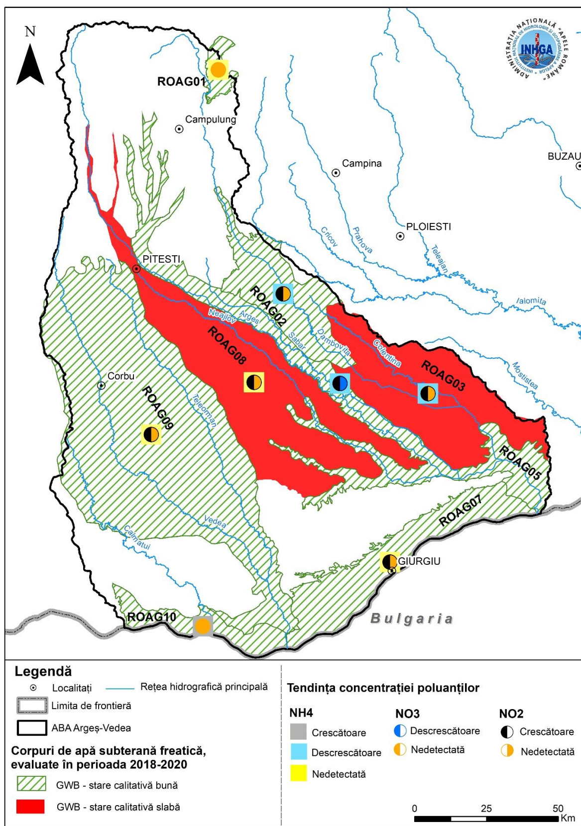
Figura 6.43. Tendințele concentrațiilor de poluanți pentru corpurile de apă subterane freatice
