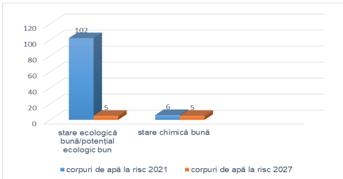
Figura 3.28. Numărul corpurilor de apă la risc din cauza presiunilor semnificative
